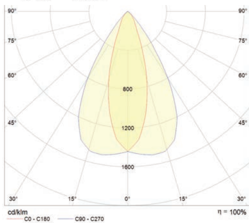
Aisle 60° x 30°
